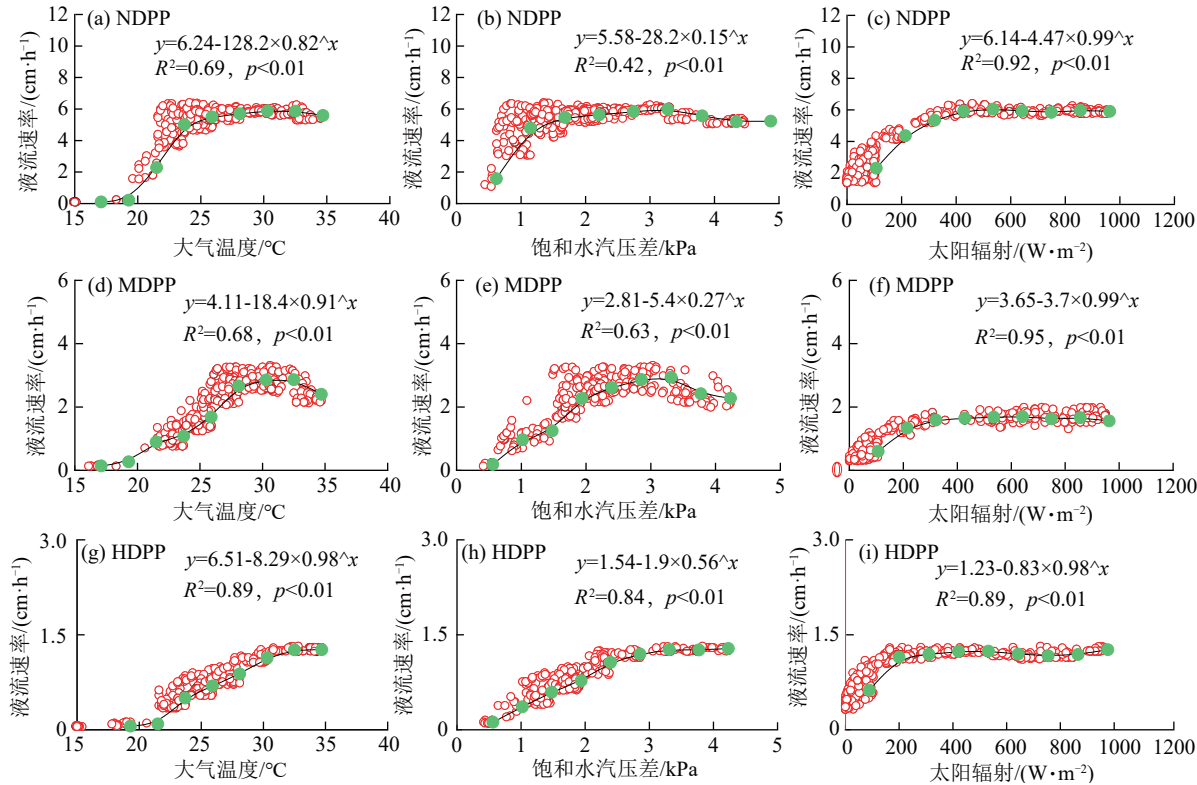
图 6 不同退化程度刺槐树干液流速率对主要气象因子响应过程的边界线分析
