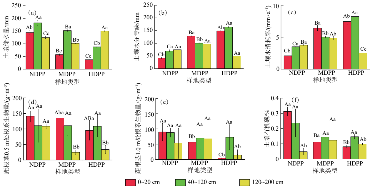
图 3 不同退化程度刺槐林地土壤水分、根系生物量、土壤有机碳变化特征
