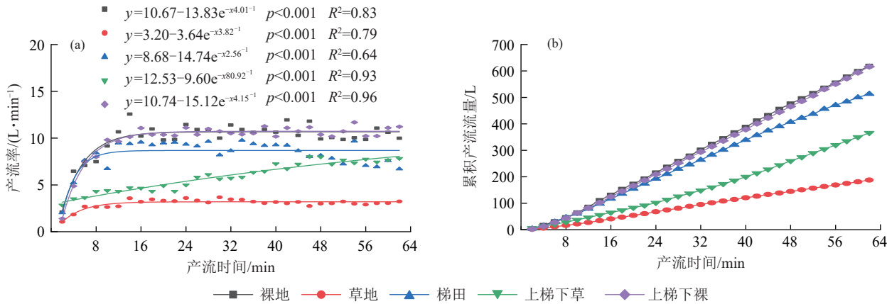
图 1 不同水土保持措施下的产流过程
