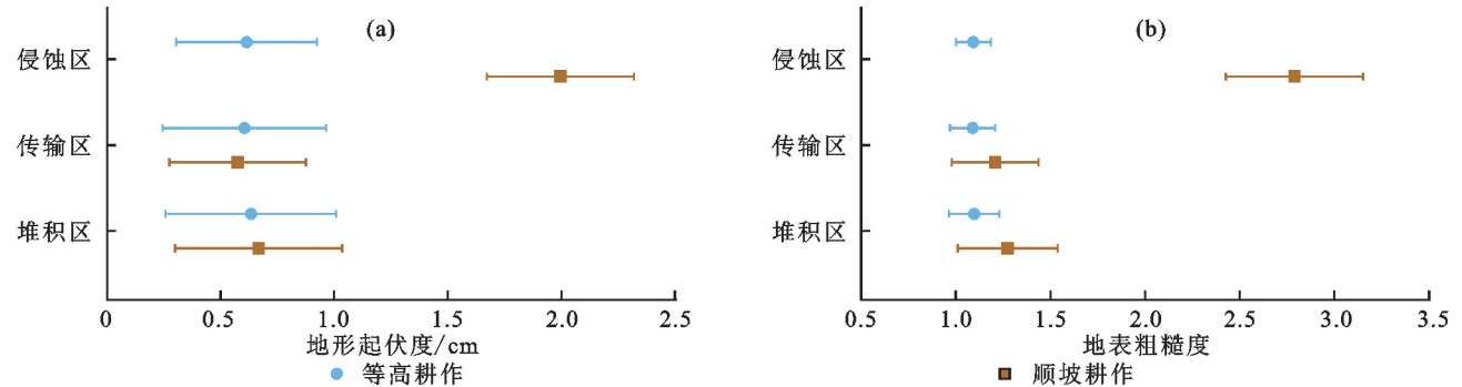
图 5 50 次耕作前后不同坡位地形起伏度与地表粗糙度的变化
