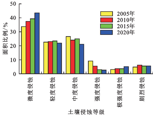
图 3 土壤侵蚀强度占比
