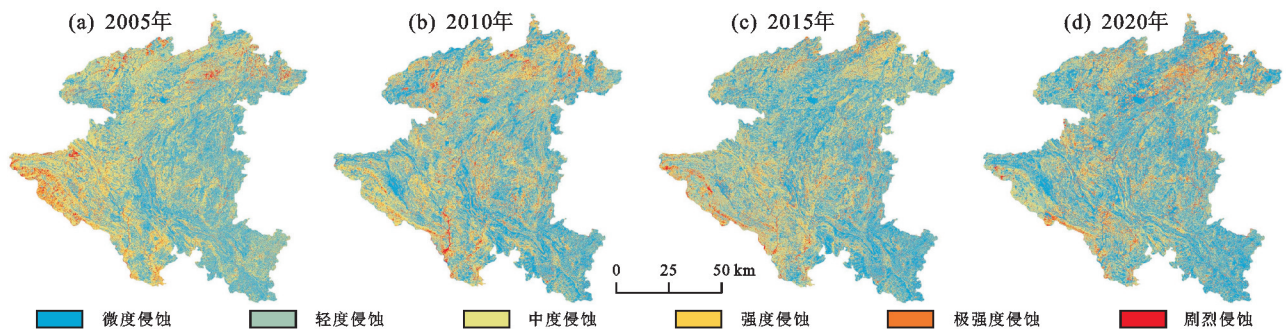
图 2 安顺市 2005—2020 年土壤侵蚀强度空间分布
