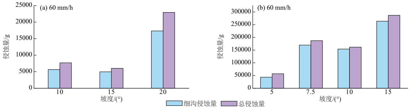
图 2 不同降雨条件下细沟侵蚀量与总侵蚀量特征
