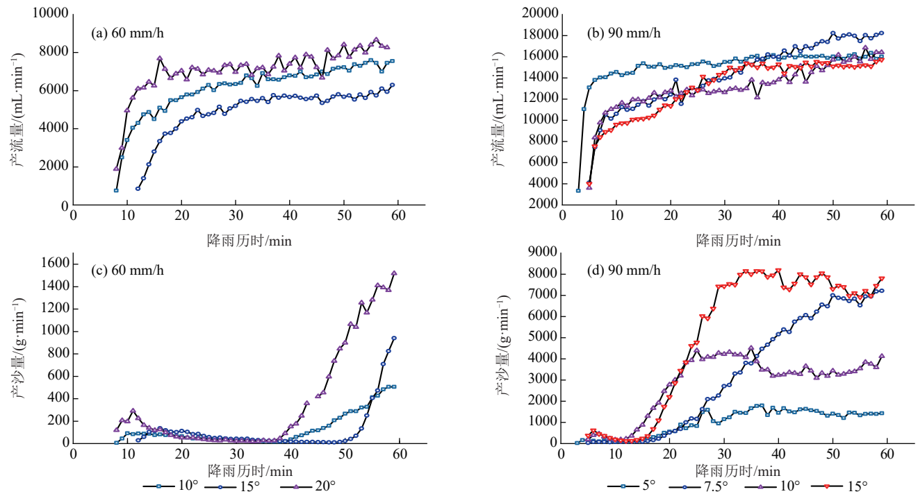
图 1 不同降雨条件下坡面产流产沙过程
