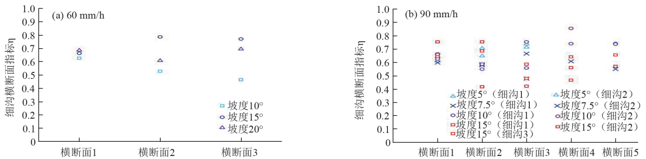
图 5 不同降雨强度与坡度条件下细沟横断面指标变化特征
