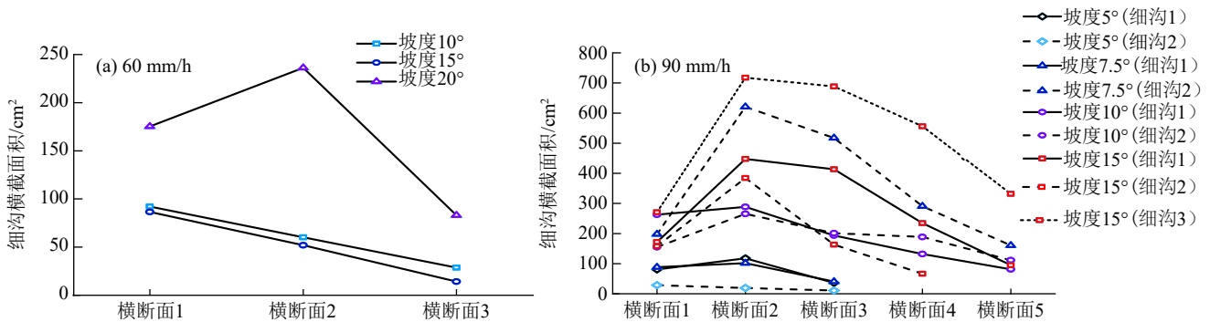
图 4 不同降雨强度与坡度条件下细沟横截面积变化特征
