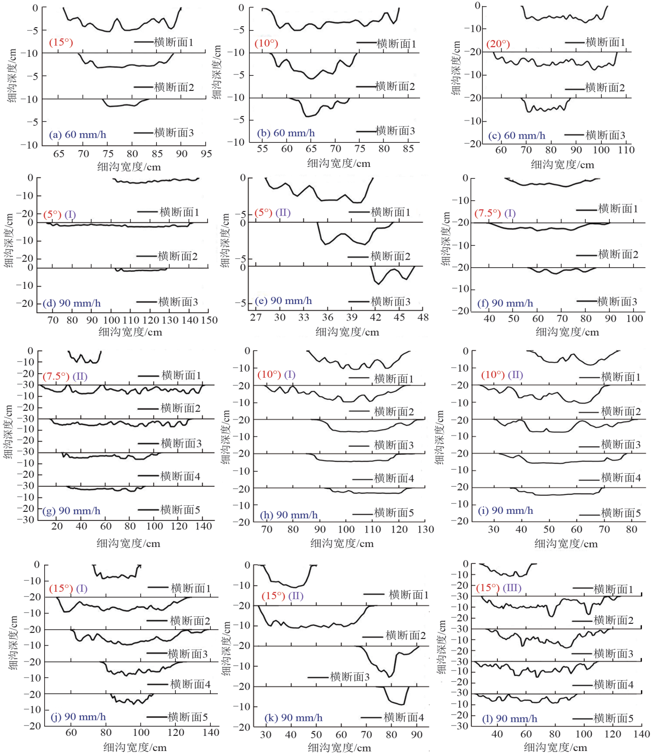
图3 细沟横断面空间分异特征
