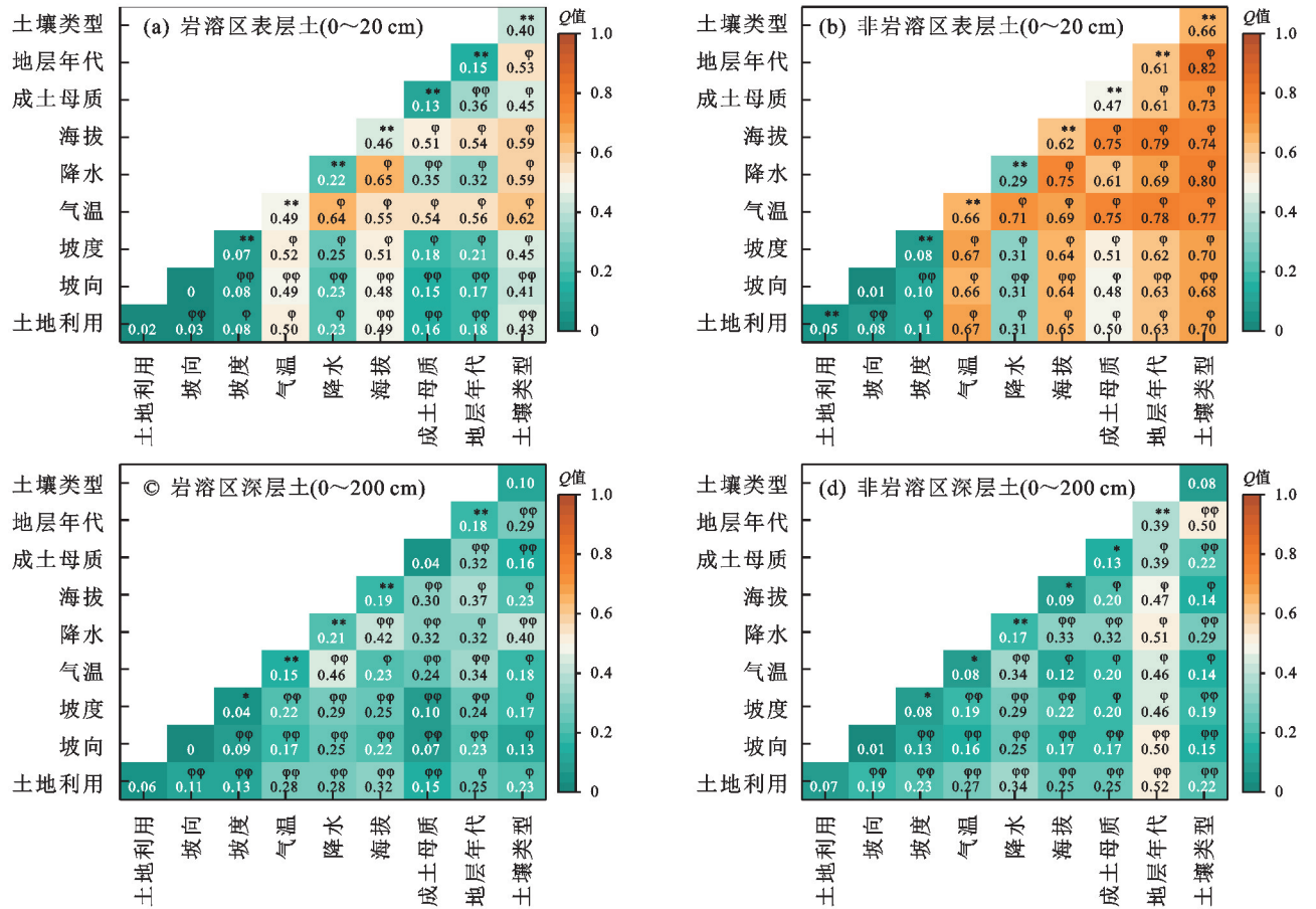
注:φ表示水平轴与垂直轴对应的两因子交互作用对 SOC 呈双因子增强影响;φφ表示非线性增强影响;* 和 ** 分别表示单因子对 SOC 的解释度在 p < 0.05 和 p < 0.01 水平显著。
