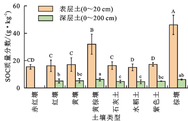
注:图柱上方不同大写和小写字母分别表示表层和深层土壤 SOC 含量在不同土壤类型间差异显著 ( p < 0.05 )。
