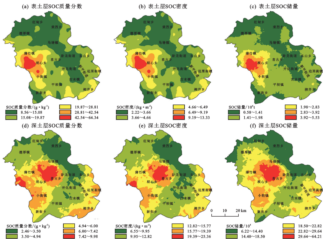
图2 文山市土壤SOC含量、密度及储量空间分布
