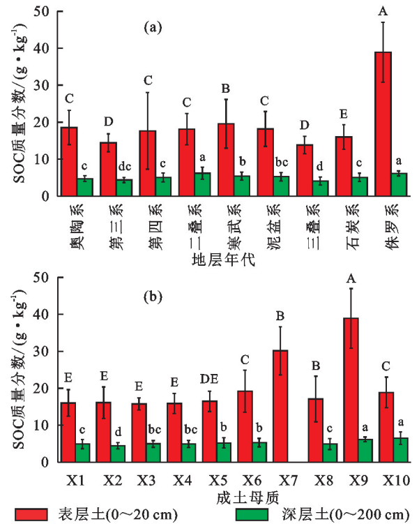
注:不同大写和小写字母分别表示表层和深层土壤 SOC 质量分数在不同地层年代或岩性间差异显著( p < 0.05 );X 1 ~X 10 分别为灰岩、白云岩、灰岩夹白云岩、灰岩与白云岩互层、白云岩夹灰岩、碳酸盐岩夹碎屑岩、碎屑岩夹碳酸盐岩、砂岩、花岗岩、玄武岩。
