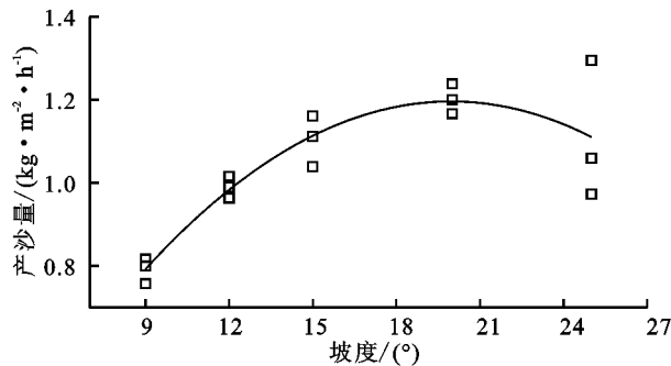
图 7 坡度与产沙量的关系
