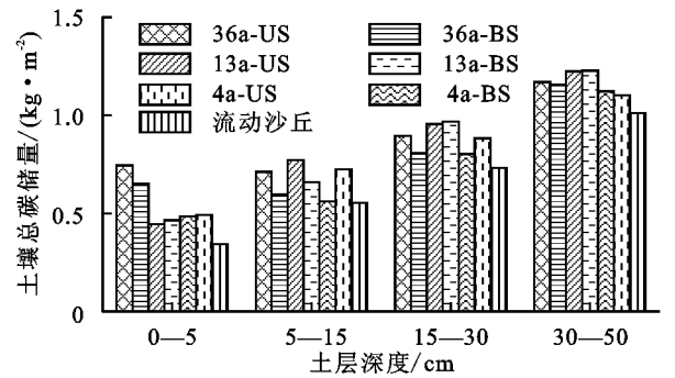
图4 民勤绿洲边缘人工梭梭林土壤总碳储量分布
